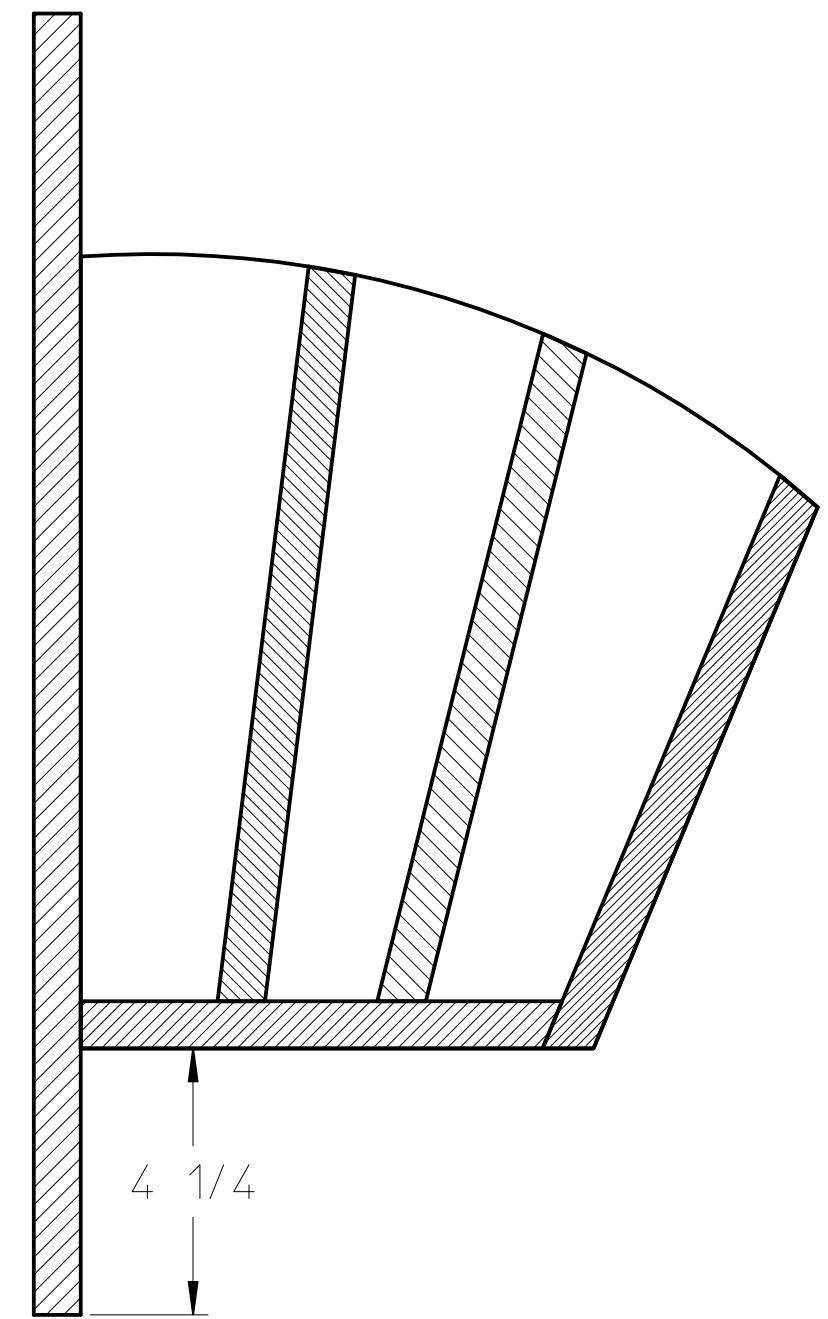
SECTION A-A SCALE 1:3
